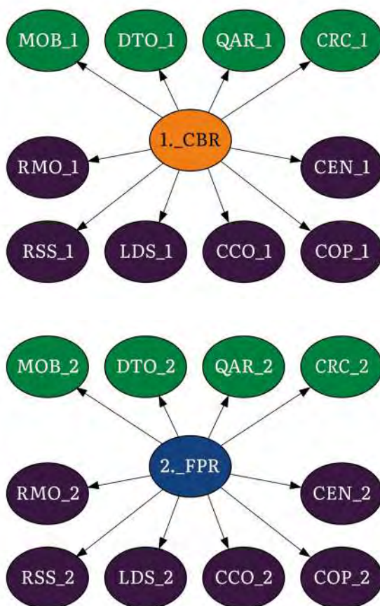
Fig 2. Red bayesiana propuesta para la selección del proceso unitario secundario.
