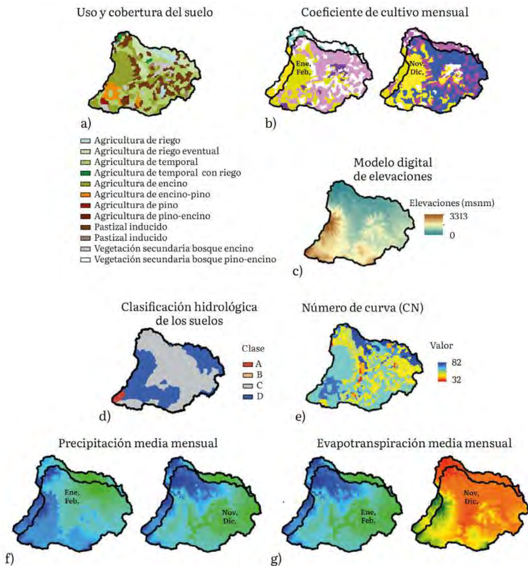
Fig. 2. Capas de entrada para estimar el rendimiento hídrico estacional: a) Clases de uso y cobertura del suelo; b) Coeficiente de cultivo mensual; c) Modelo digital de elevaciones; d) Clasificación hidrológica de los suelos; e) Número de la curva; f) Precipitación media mensual; g) Evapotranspiración de referencia mensual [20].
