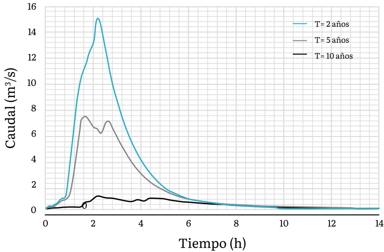
Fig. 6. Hidrogramas de salida en la cuenca tributaria.
