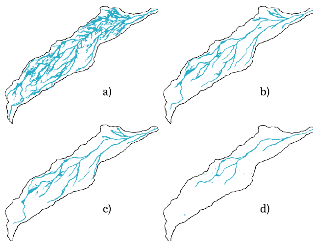
Fig. 5. Simulación del Proceso Lluvia – Esguerrimiento evento asociado a un T_r = 10 Años. a) t=4.0 h; b) t=5.0 h; c) t=6.0 h; d) t=7.0 h.
