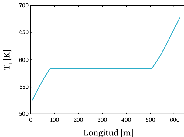
Fig. 6. Temperatura del agua/vapor a lo largo de un lazo de reflectores Fresnel [4], [36].
