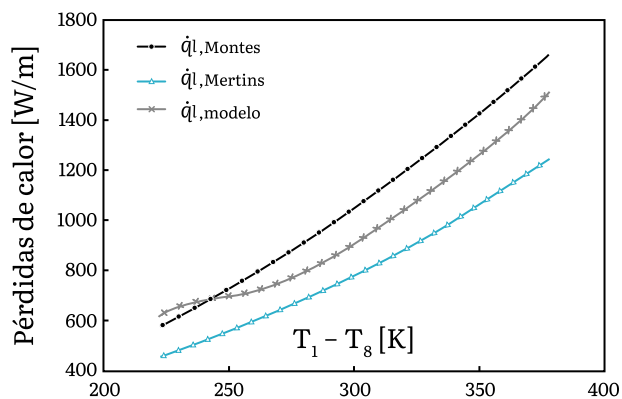
Fig. 4. Comparativa de las pérdidas térmicas del modelo [21] contra el modelo de Montes [4] y Mertins [36].
