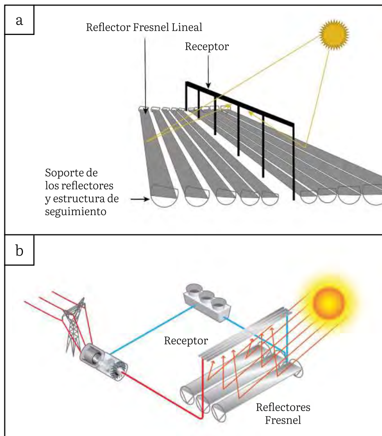
Fig. 2. Esquemático de los sistemas Fresnel. a) Configuración de un módulo [13]; b) Configuración de una planta solar con LFR [14].
