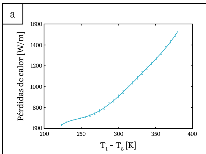
Fig. 5. Barras de error. (a) Comparación con el modelo de Montes [4]; (b) Comparación con el modelo de Mertins [36].
