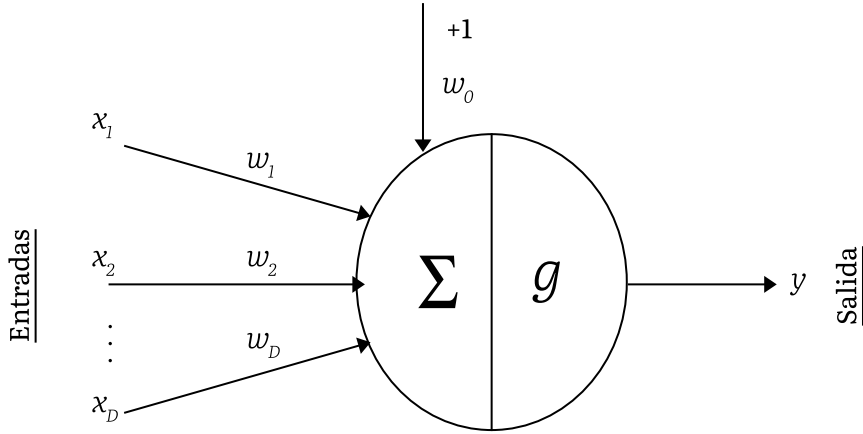
Fig. 2. Modelo de neurona propuesto por McCulloh y Pitts.
