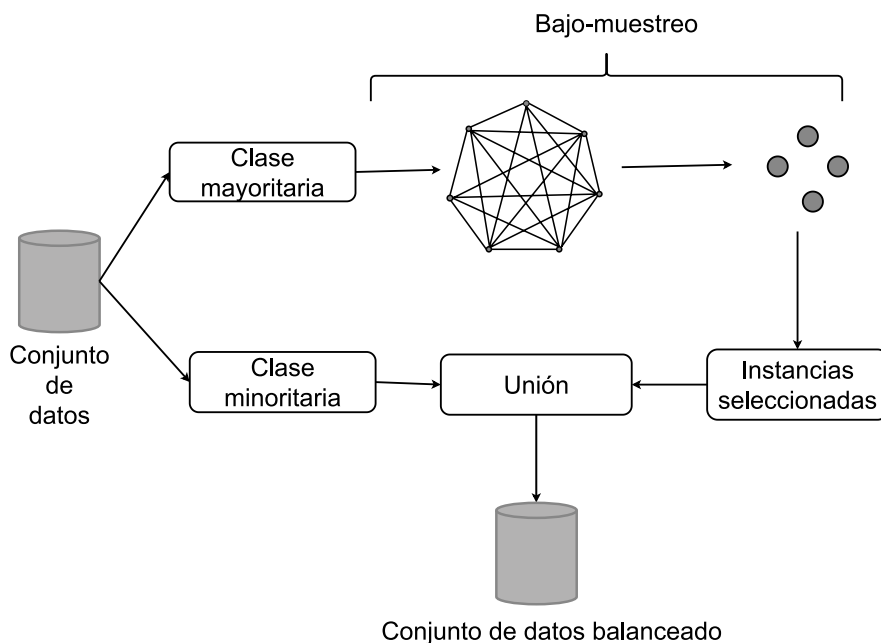
Fig. 4. Flujo de trabajo de algoritmos basados en grafos.
