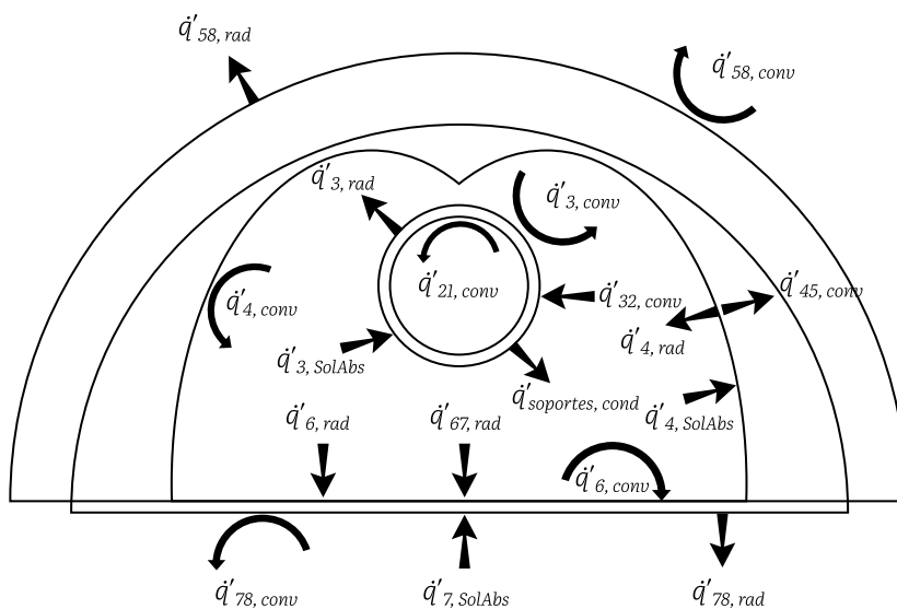
Fig. 3. Flujos de calor en el receptor [21].
