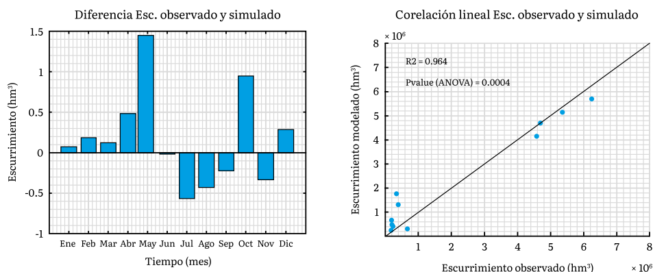
Fig 3. a) Diferencia entre los volúmenes medios medidos por la estación hidrométrica y los obtenidos por el modelo; b) Correlación entre el escurrimiento observado y modelado.
